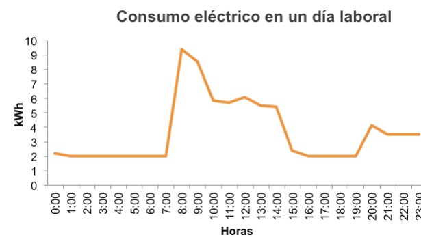
Gráfico 8. Ejemplo de resultado gráfico obtenido con un analizador de redes en una oficina.
