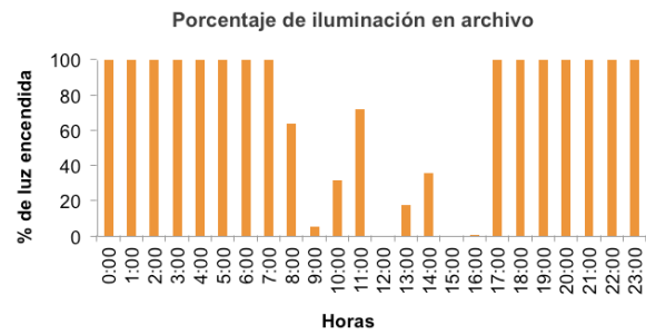
Gráfico 10. Ejemplo de resultado gráfico obtenido con un registrador de ocupación.
