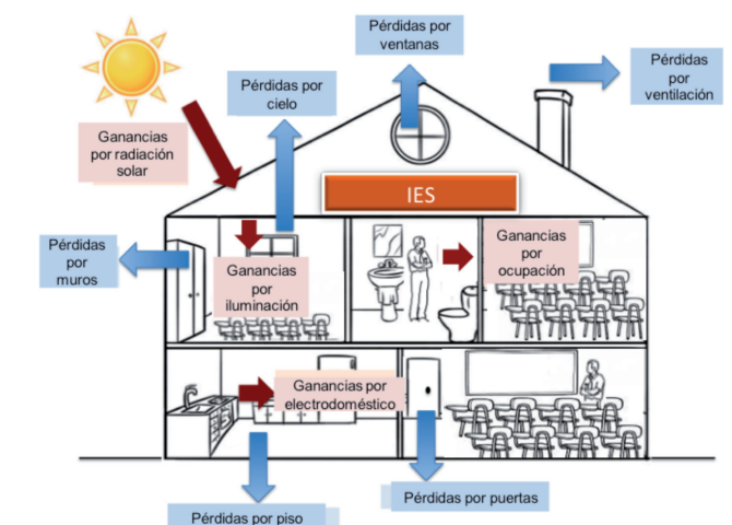
Figura 5. Pérdidas y ganancias de calor y refrigeración en un edificio.
