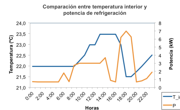
Gráfico 9. Ejemplo de resultado gráfico obtenido con un registrador de temperatura.
